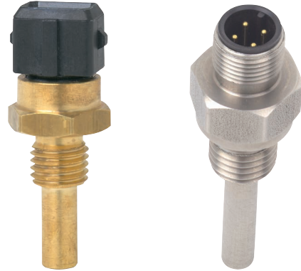
Abb. links: Stecker AMP Junior Power Timer Abb. rechts: Rundstecker M12 x 1
